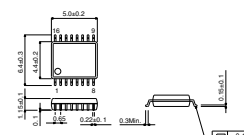
SSOP-B16
